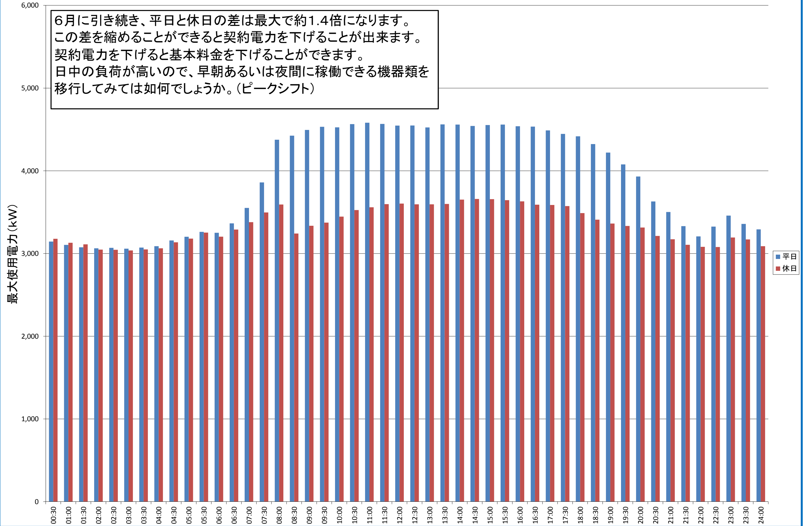
本荘北キャンパス 7月の時間帯別最大使用電力平均値
