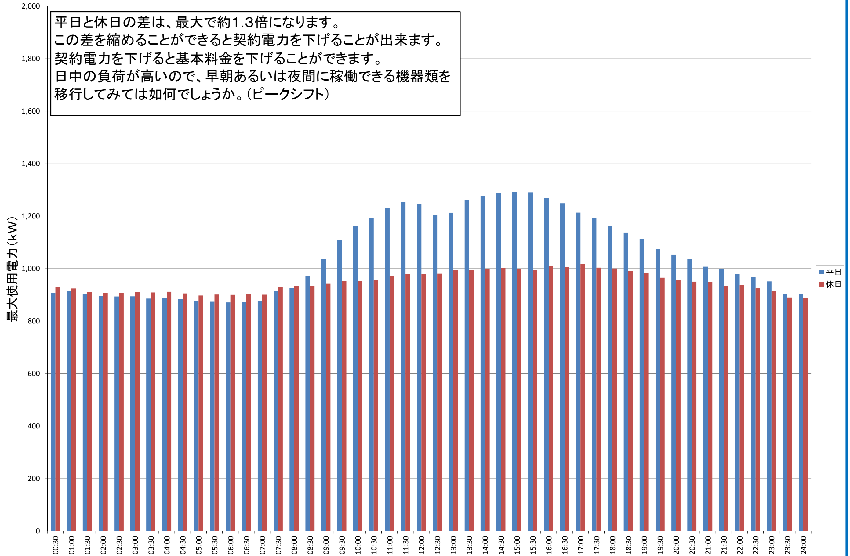
本荘中キャンパス 6月の時間帯別最大使用電力平均値
